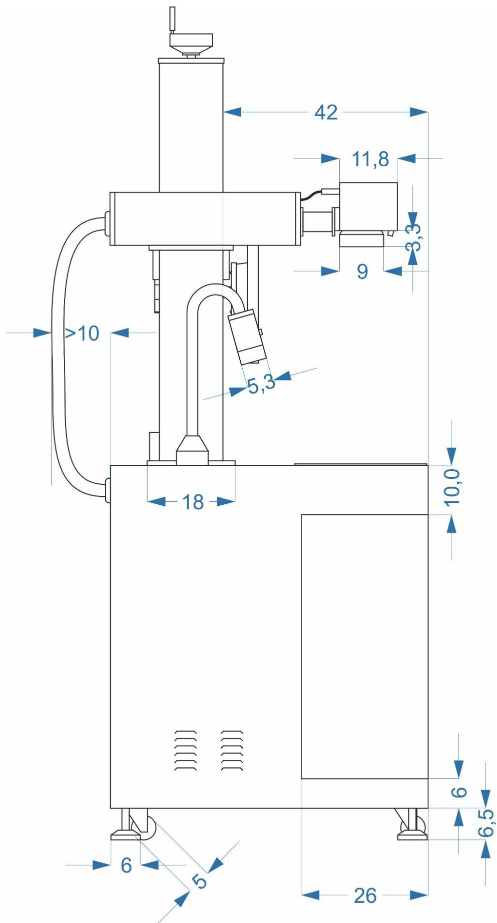
Рис. 3. Вид слева.
