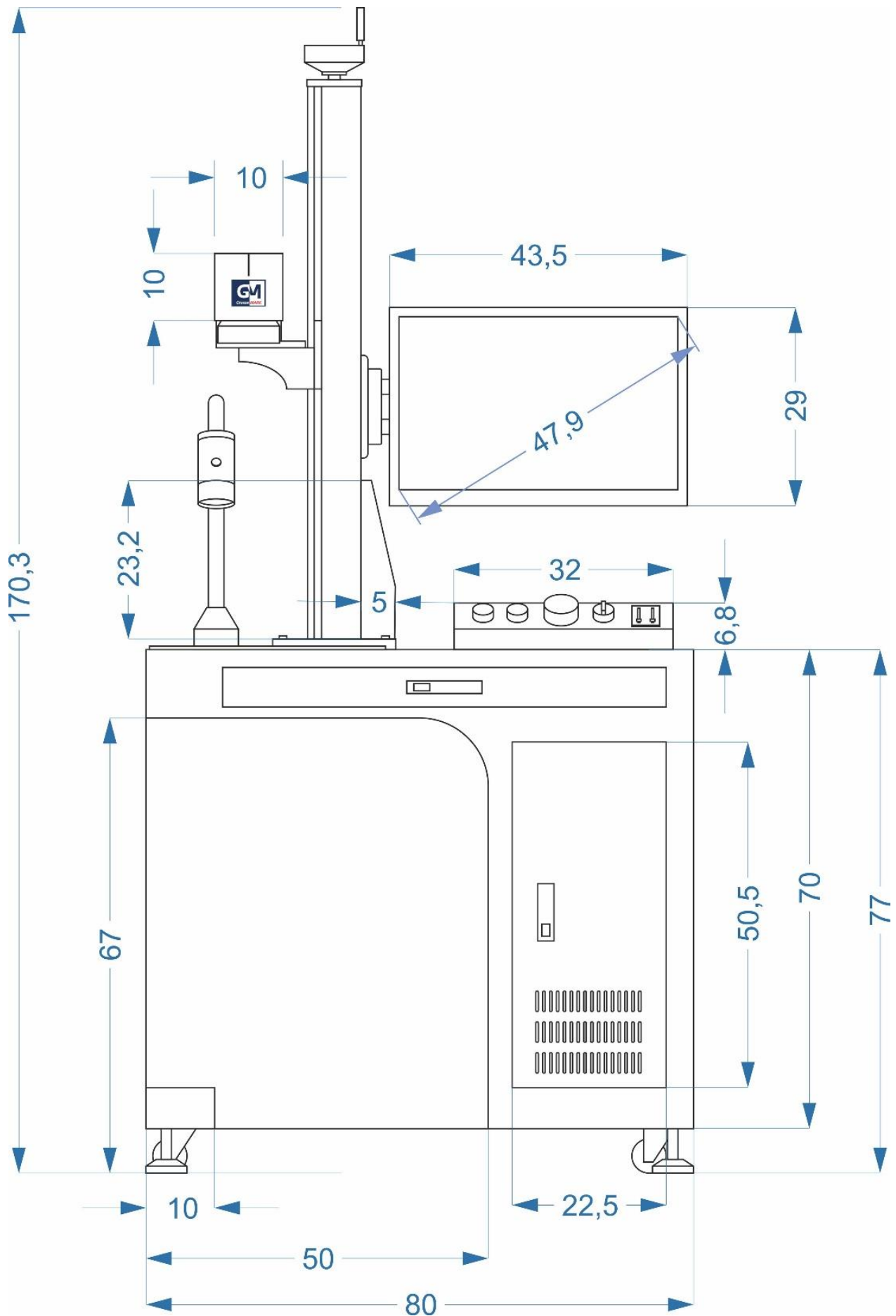
Рис. 2. Вид спереди.
