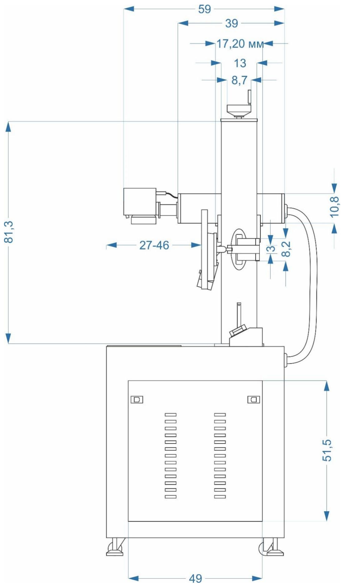
Рис. 1. Вид справа.
