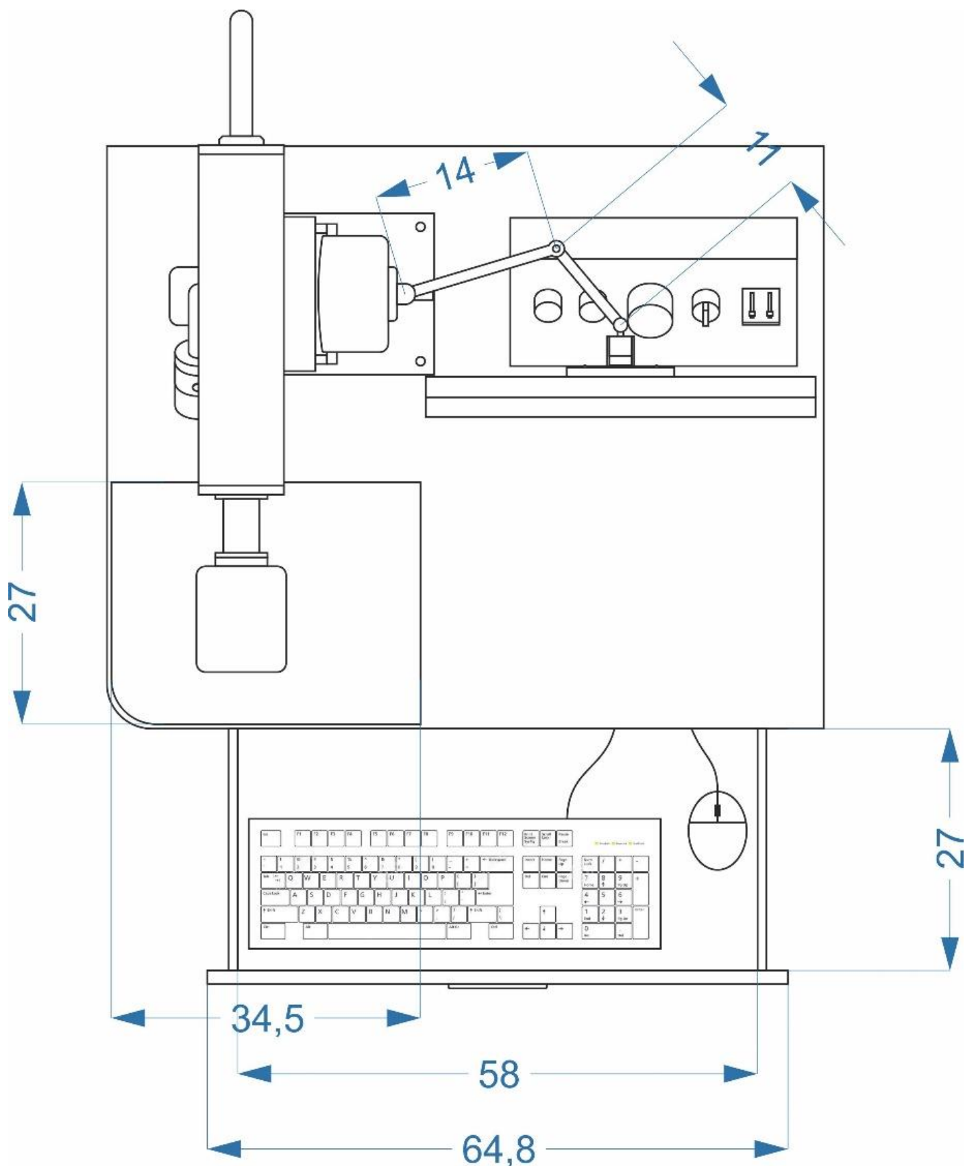
Рис. 4. Вид сверху.
